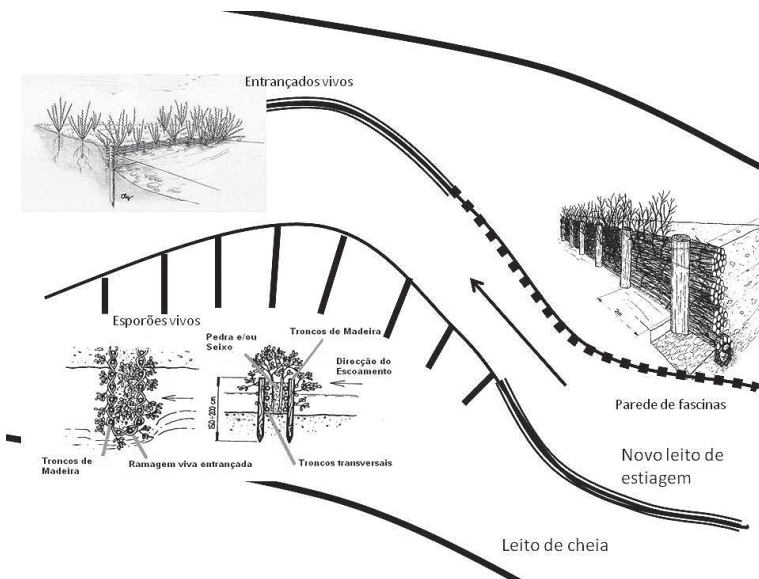
Fig. 4.17. Ilustração hipotética de uma intervenção de reconstrução dum leito de estiagem num leito de cheia morfologicamente indiferenciado devido a uma gestão desadequada
