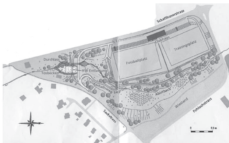
Fig. 4.24. Exemplo de uma bacia de retenção (Forloch Martalen, Zurique) cujo espaço de retenção corresponde às instalações de um clube de futebol (dois campos relvados com bancadas e instalações de apoio nos taludes marginais e no coroamento, respectivamente) e uma zona verde. Nenhum dos usos dentro da bacia é incompatível com uma submersão curta e durante todo o ano preenchem serviços sociais do maior interesse. A zona dos campos de futebol nunca é inundado por cheias com tempo de retorno (TR) de até 5 anos e o campo principal apenas será submerso por cheias com TR superior a 10 anos. A Bacia está dimensionada para cheias com TR até 200 anos.
