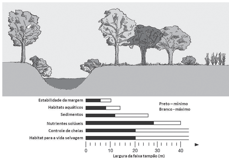
Fig. 3.8. Ilustração das diferentes funções asseguradas pela vegetação ripícola e das dimensões mínimas exigidas para o pleno preenchimento dessas funções (adaptado de RIPARIA, 2005)
