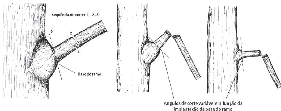
Fig. 4.12. Sequência do corte de um ramo de modo a evitar a formação de rachas ou outras feridas: cortes preparatórios 1 e 2 para garantir que o ramo ao partir não "rasga" o tronco, 3 - corte definitivo do toco remanescente, de modo a garantir a menor superfície de corte possível (Florineth, 2004).
