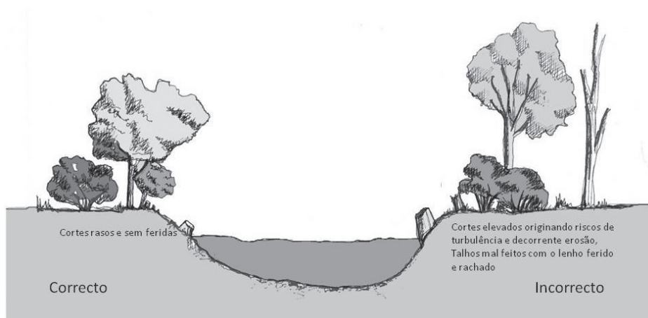
Fig. 4.13. Exemplo de um processo de limpeza de grandes árvores correcta e incorrectamente conduzidos (adaptado de Jund et al. 2000)
