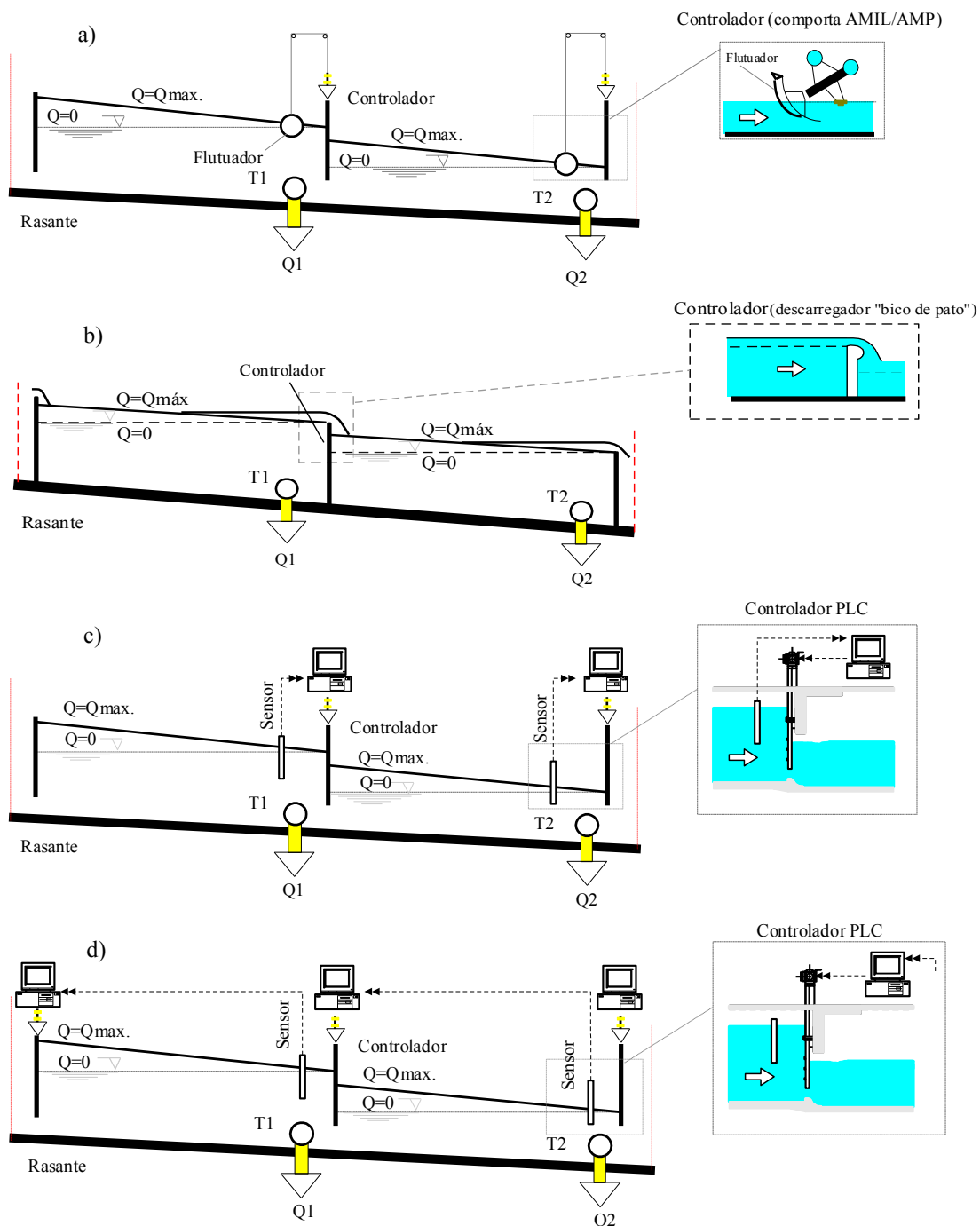
Figura 1. Controle local por montante e controle por jusante à distância (Rijo, 2008).
