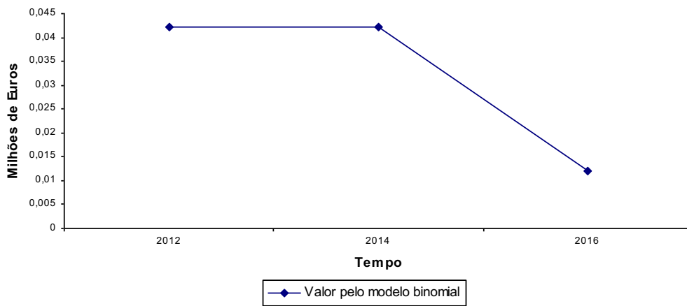
Figura 2 Evolução do valor pelo Modelo Binomial
