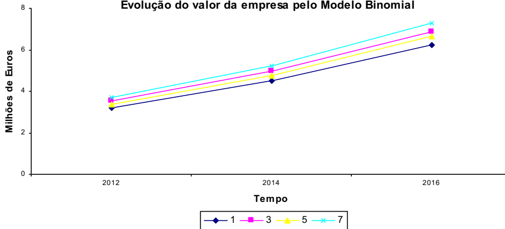
Figura 3 Evolução do valor da empresa pelo Modelo Binomial
