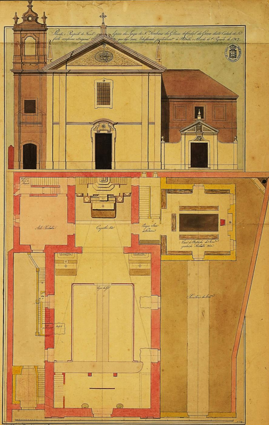
PEREIRA, Luís Gonzaga, 1796-1868 [Planta e alçado da fachada da igreja de Nossa Senhora da Glória do Cardal da Graça] 1826 Fonte: BNP.
