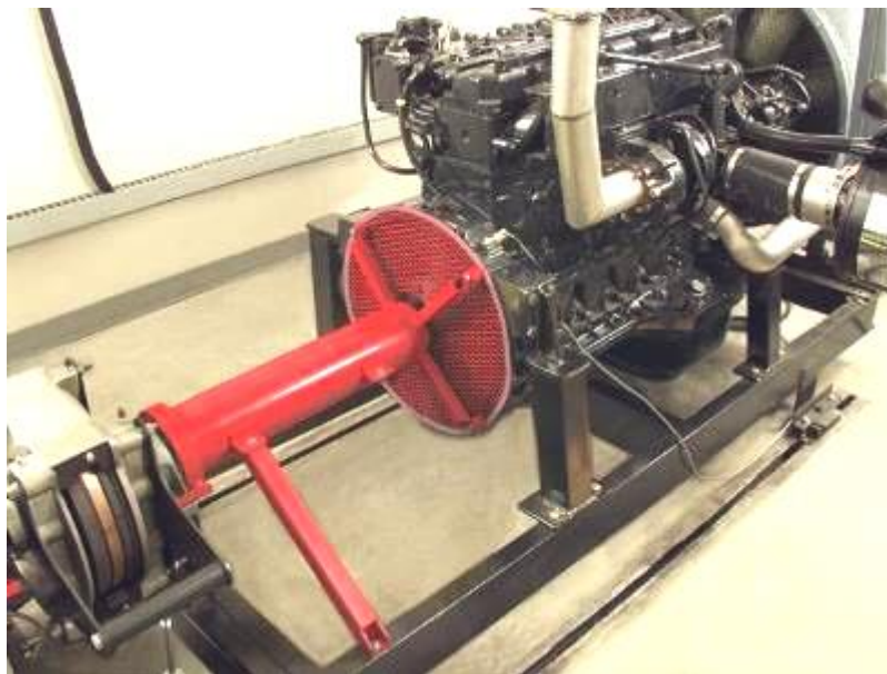
Ensaio de um motor Diesel (à direita) num freio dinamométrico (à esquerda)
