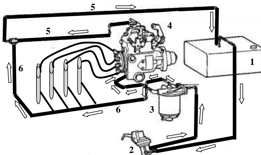
Circuito de Baixa Pressão
