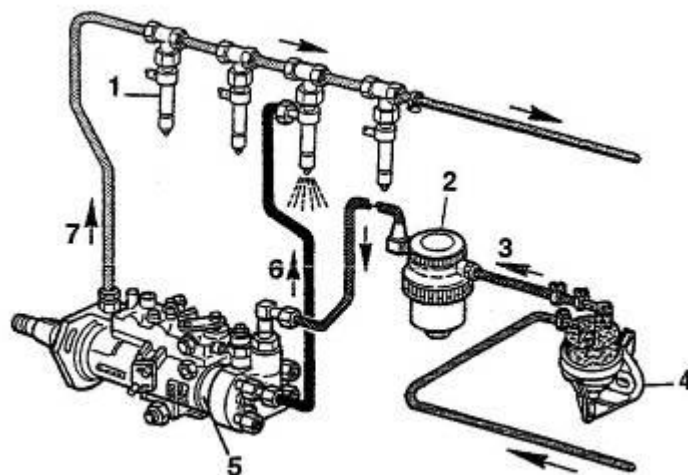
Sistema de injeção do Tractor John Deere 4045 DRT 1 - Injector; 2 - Filtro de combustível; 3 - Conduto de baixa pressão; 4 - Bomba de alimentação (de membrana); 5 - Bomba de injeção (tipo distribuidor); 6 - Tubo de alta pressão; 7 - Retorno de gasóleo ao depósito.
