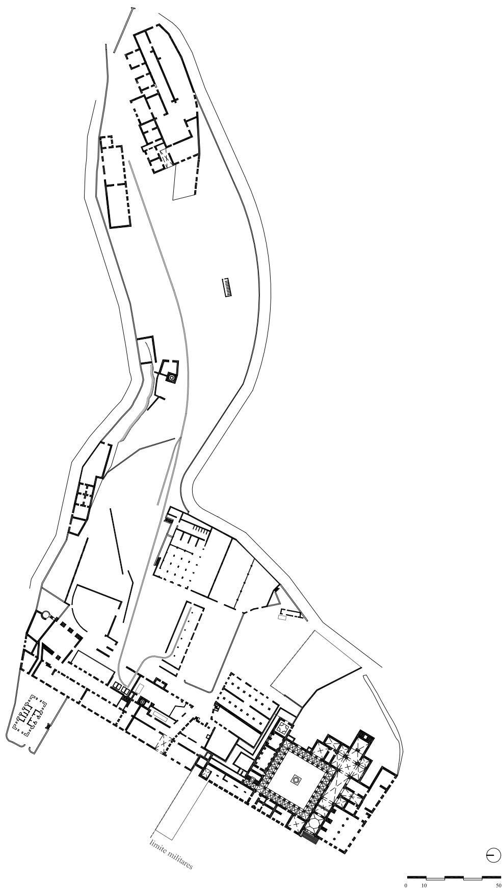
Fig. I-e - Planta da Fábrica Robinson em Portalegre-1927. Portugal
