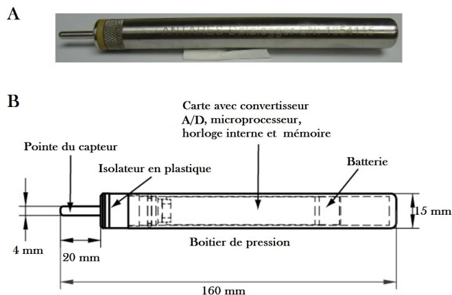
Figure 6. A : Enregistreur de la température (Miniaturized Temperature data Logger (MTL)), B : schéma détaillé d'un MTL (Pfender &Villinger 2002), A/D = analogique-au-digital.
