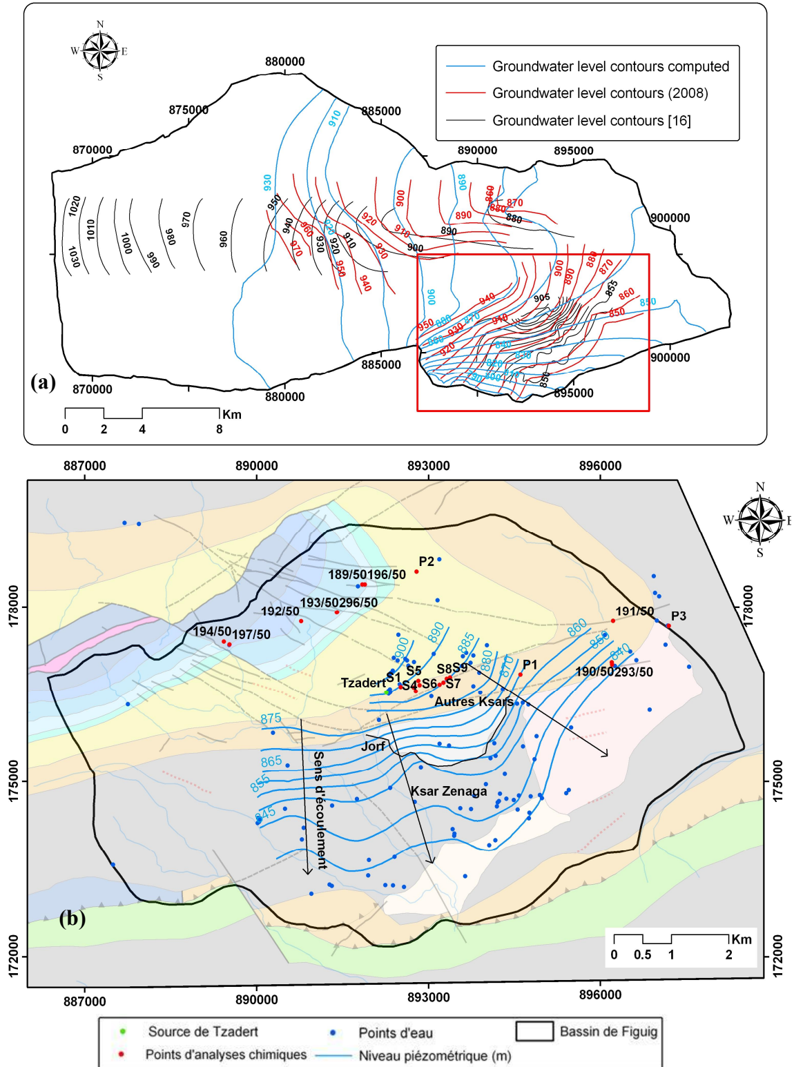
Figure 3. Carte piézométrique de l'année 2010: (a) Plaines Tisserfine, Arja et Figuig (Jilali 2014b) , (b) Figuig. Figure 3. Map of piezometric 2010: (a) Tisserfine Plains, Arja and Figuig (Jilali 2014b), (b) Figuig.
