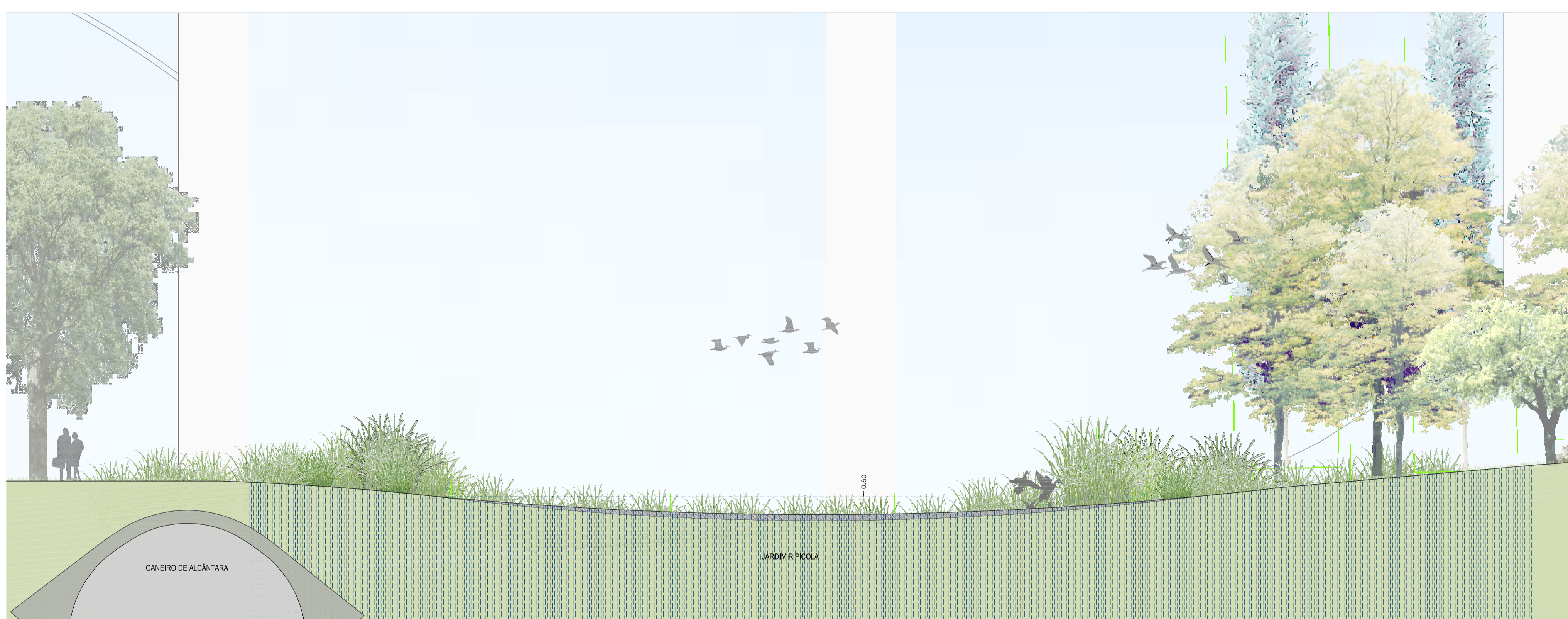
CORTE TIPO - JARDIM URBANO
