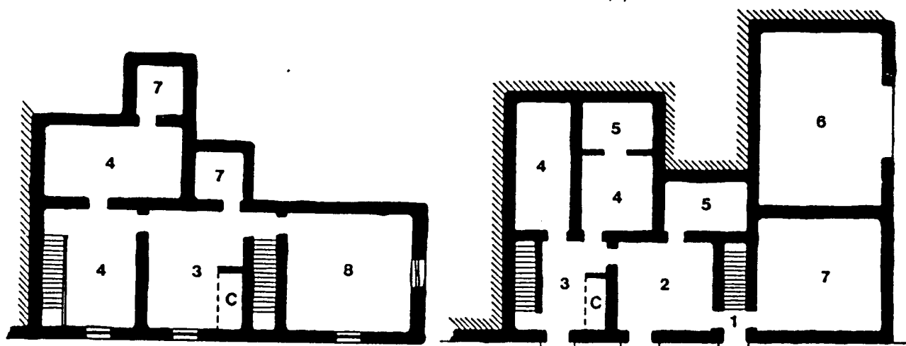
FIGURA Nº II.2. - PLANTAS DE CASAS URBANAS TRANSFERIDAS PARA UMA LOCALIDADE RURAL DO ALTO ALENTEJO (1)
