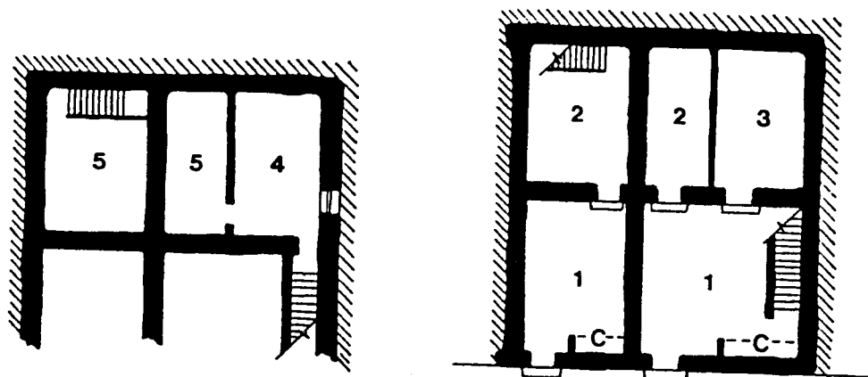
FIGURA Nº II.1. - PLANTAS DE CASAS TRADICIONAIS DE UMA LOCALIDADE RURAL DO ALTO ALENTEJO (1)
