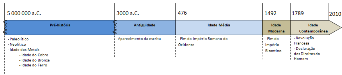
Fig. 2. Línea de tiempo: prehistoria y períodos de la historia.
