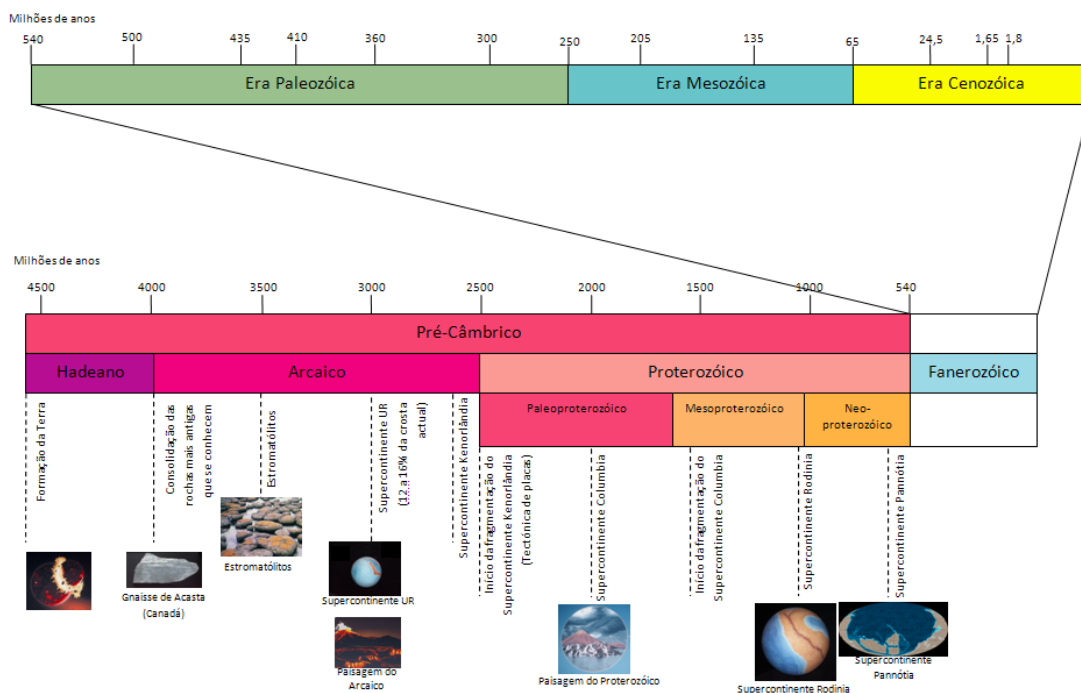
Fig. 3. Escala de tiempo geológico.
