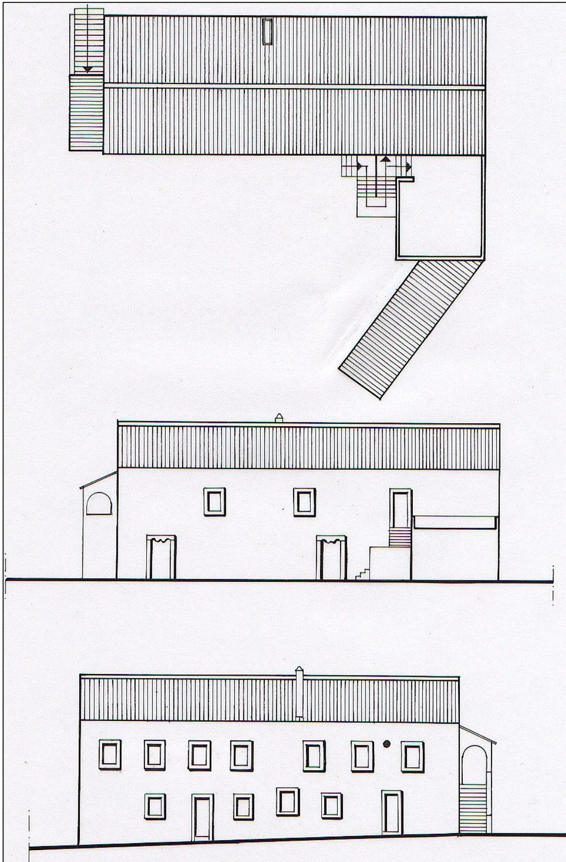
Fig. 10 – Turquel. Quinta da Granja, planta do edifício de habitação. Esc.1/200
