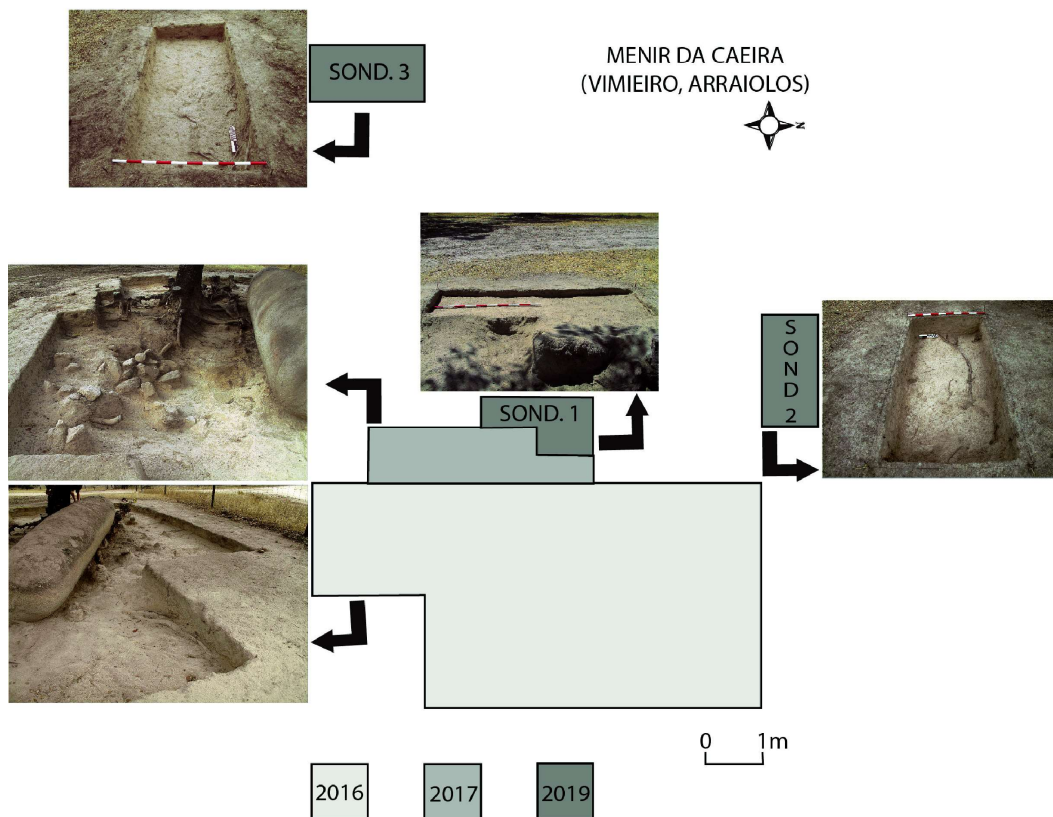
Fig. 4. Planta geral com indicação das áreas intervencionadas, por ano
