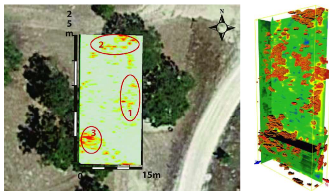
Fig. 9. Resultados da prospeção geofísica realizada em 2019
