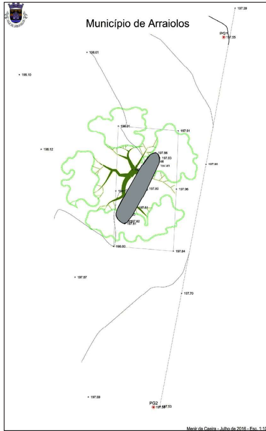
Fig. 5. Levantamento topográfico realizado pelos Serviços Técnicos da autarquia de Arraiolos
