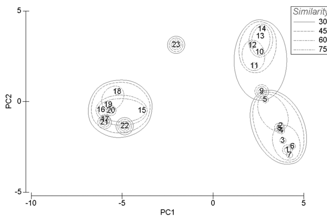
Fig. 3 - Ordination diagram (PCA).
