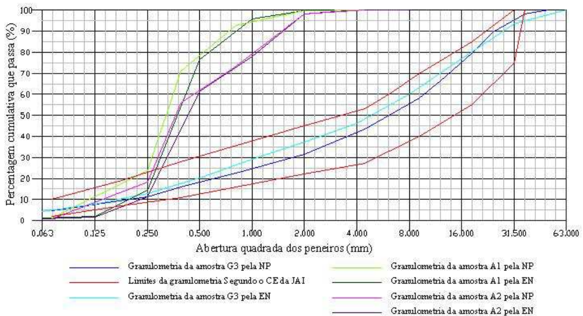
Gráfico A2.2 – Gráfico de representação das curvas granulométricas, segundo a norma Europeia, com todas as curvas das amostras analisadas e com a representação do fuso granulométrico B retirada do CETO198.
