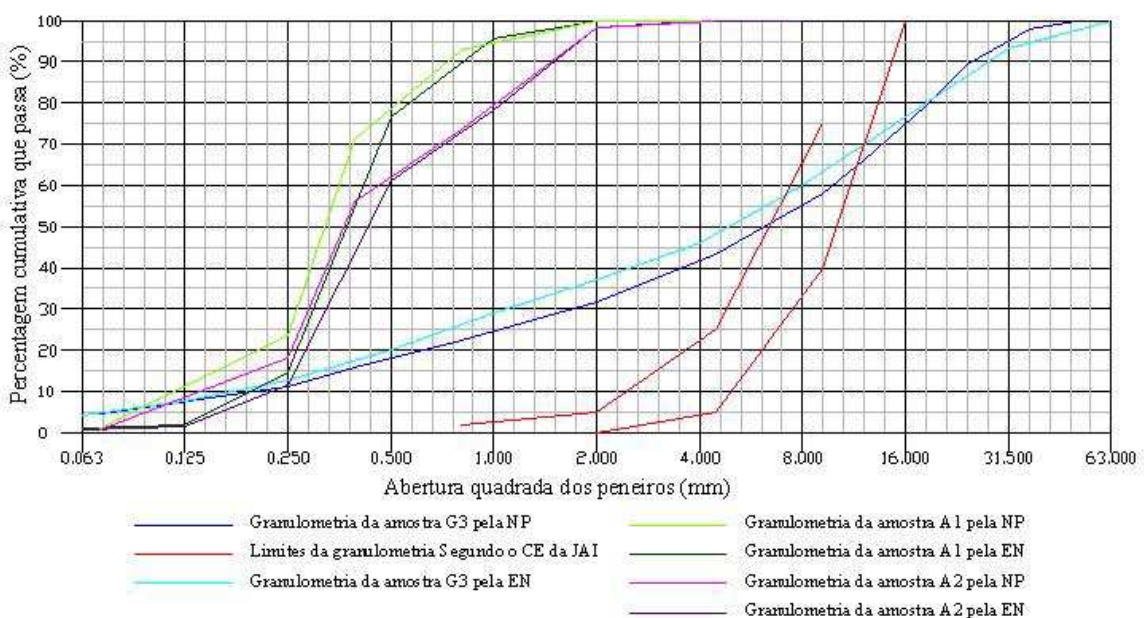
Gráfico A2.10 – Gráfico de representação das curvas granulométricas, segundo a norma Europeia, com todas as curvas das amostras analisadas e com a representação do fuso granulométrico J retirada do CETO198.
