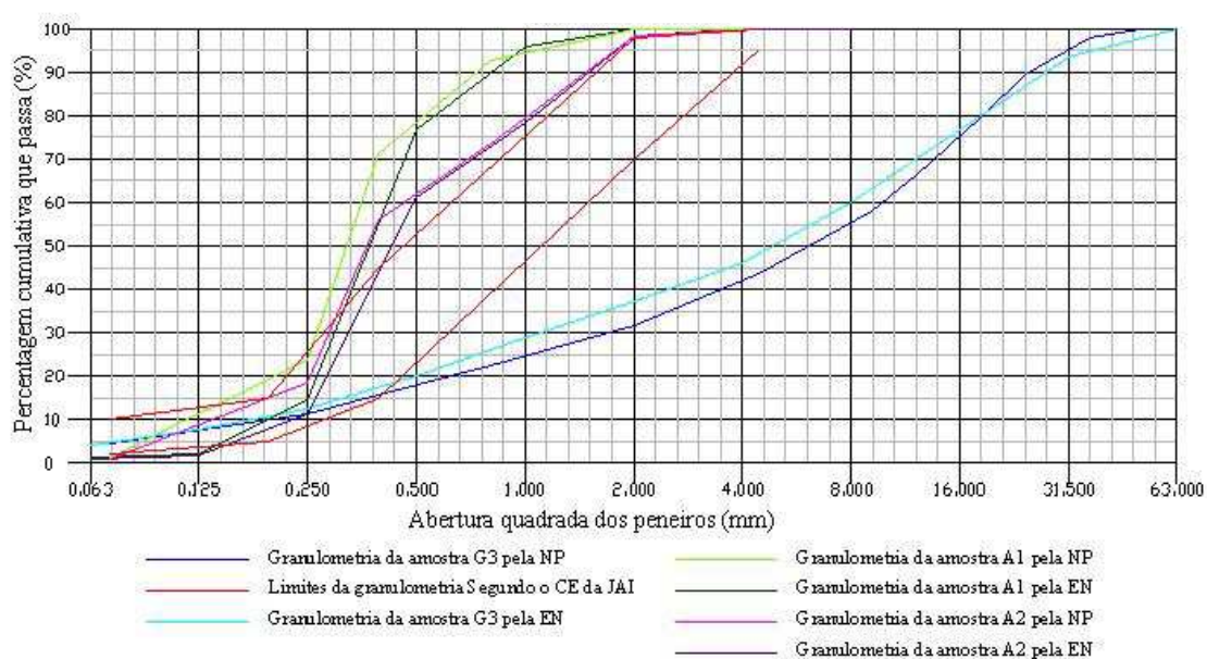
Gráfico A2.3 – Gráfico de representação das curvas granulométricas, segundo a norma Europeia, com todas as curvas das amostras analisadas e com a representação do fuso granulométrico C retirada do CETO198.
