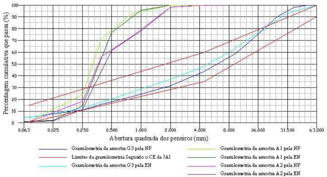
Gráfico A2.1 – Gráfico de representação das curvas granulométricas, segundo a norma Europeia, com todas as curvas das amostras analisadas e com a representação do fuso granulométrico A retirada do CETO198.
