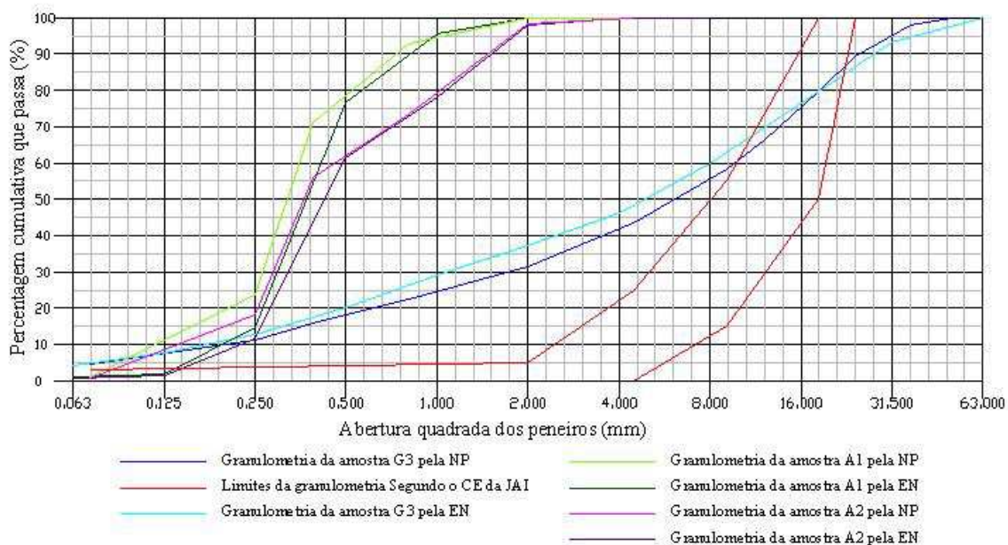
Gráfico A2.4 – Gráfico de representação das curvas granulométricas, segundo a norma Europeia, com todas as curvas das amostras analisadas e com a representação do fuso granulométrico D retirada do CETO198.
