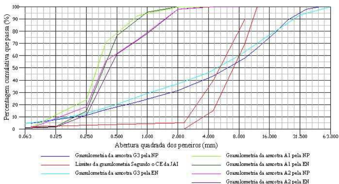
Gráfico A2.6 – Gráfico de representação das curvas granulométricas, segundo a norma Europeia, com todas as curvas das amostras analisadas e com a representação do fuso granulométrico F retirada do CETO198.
