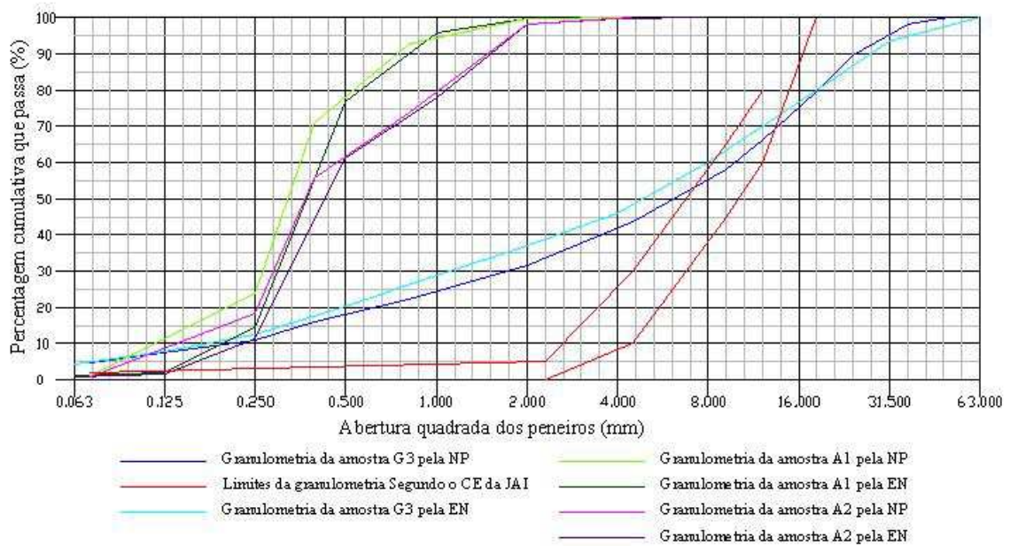
Gráfico A2.7 – Gráfico de representação das curvas granulométricas, segundo a norma Europeia, com todas as curvas das amostras analisadas e com a representação do fuso granulométrico G retirada do CETO198.
