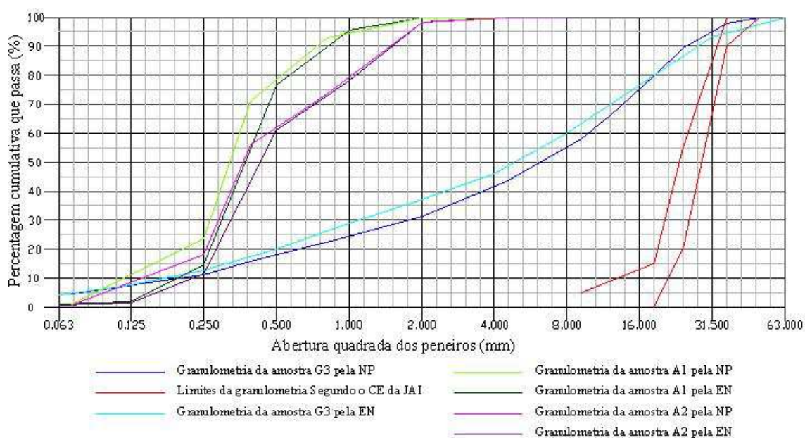
Gráfico A2.9 – Gráfico de representação das curvas granulométricas, segundo a norma Europeia, com todas as curvas das amostras analisadas e com a representação do fuso granulométrico I retirada do CETO198.
