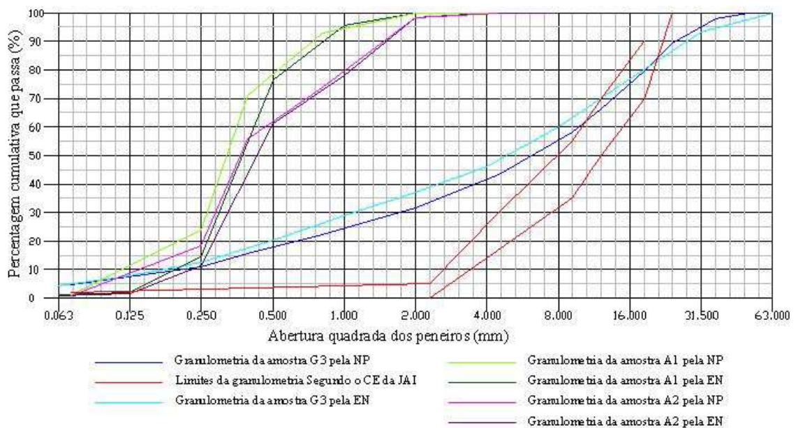
Gráfico A2.8 – Gráfico de representação das curvas granulométricas, segundo a norma Europeia, com todas as curvas das amostras analisadas e com a representação do fuso granulométrico H retirada do CETO198.
