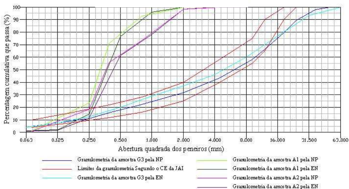
Gráfico A2.5 – Gráfico de representação das curvas granulométricas, segundo a norma Europeia, com todas as curvas das amostras analisadas e com a representação do fuso granulométrico E retirada do CETO198.
