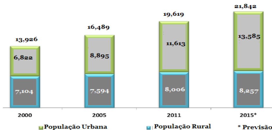
Figura 3 – População de Angola 2000-2015 (milhares de pessoas)
