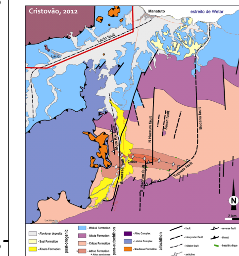
LEGENDA Formação de Aileu Formação de Wailuli Formação de Maubisse Aluviões
