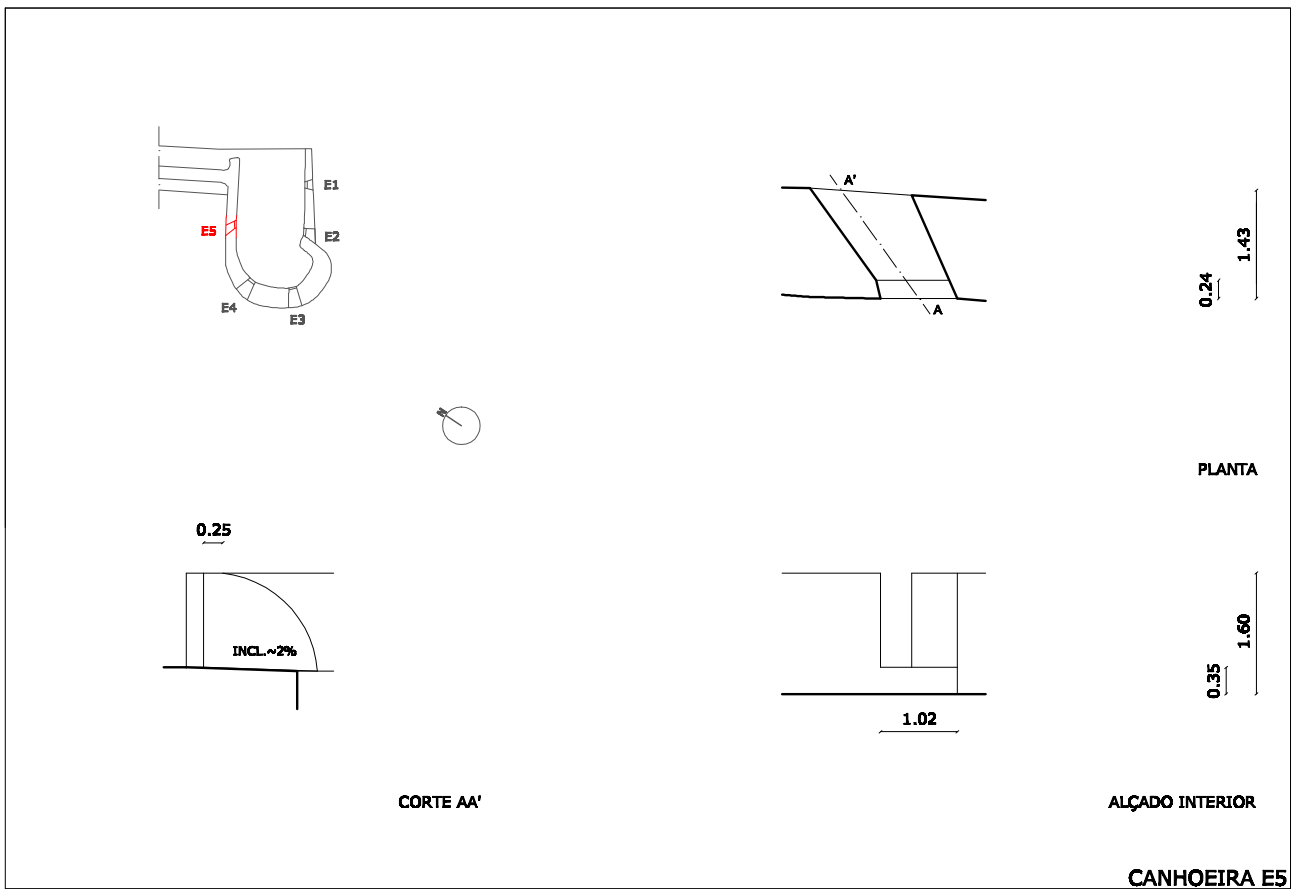
DESENHO 32 - FORTALEZA DE DIU
