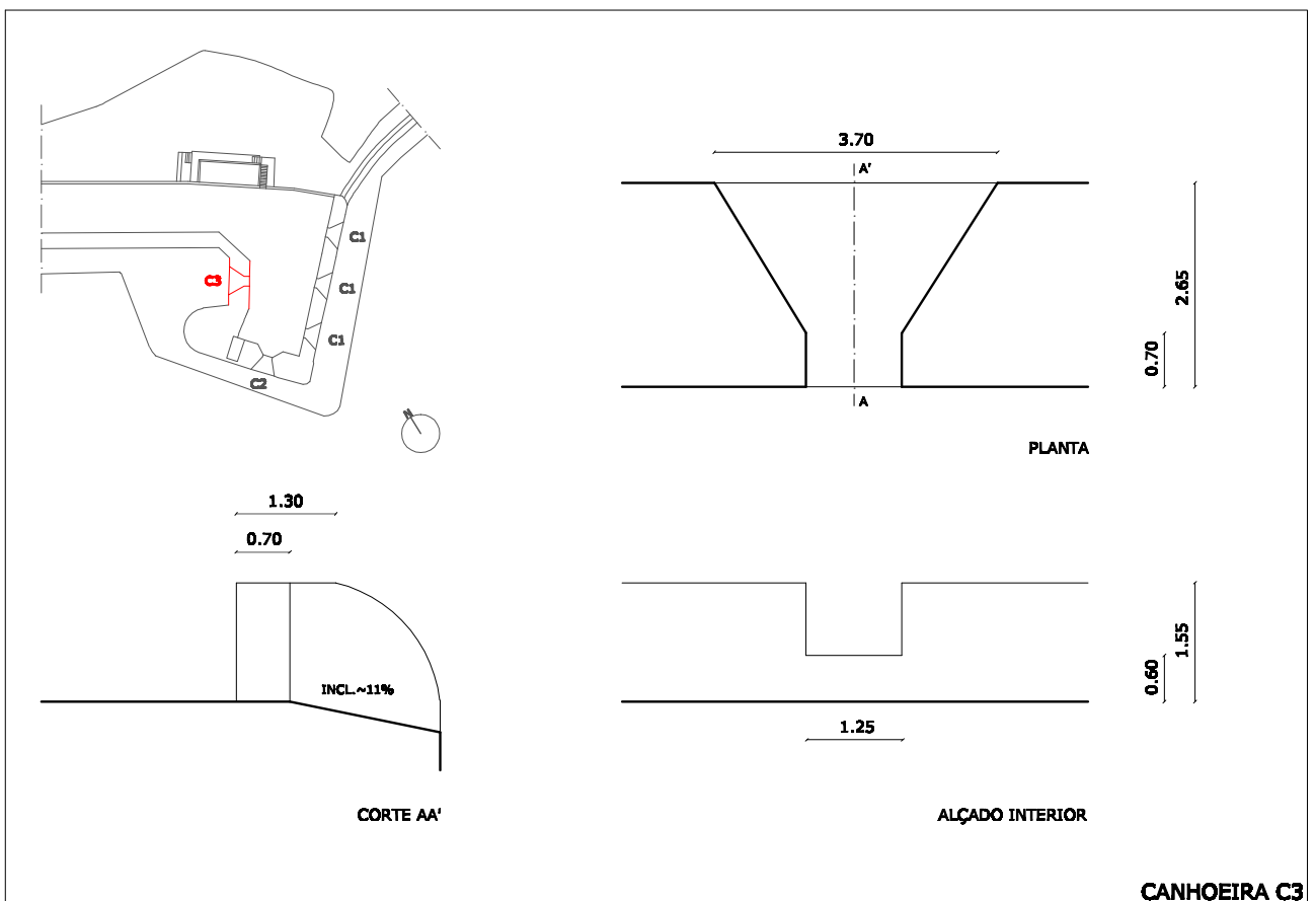
DESENHO 20 - FORTALEZA DE DIU
